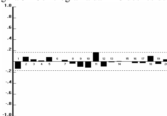
Figura 3 - Correlograma da FAC dos resíduos.
