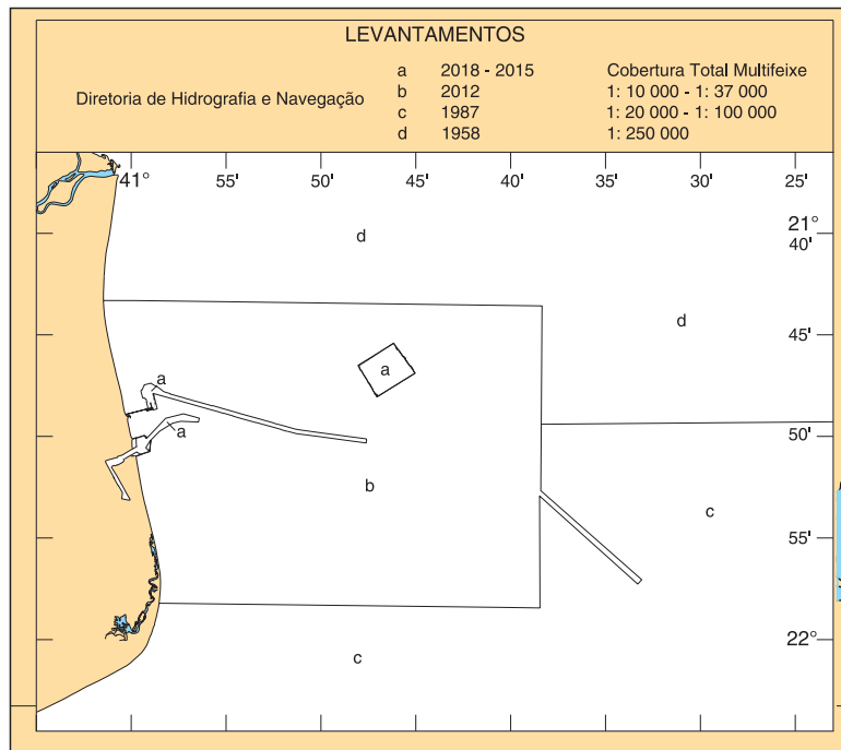
Block for Chart 1406 - 2 nd EDITION. Correção para a Carta 1406 - 2 a EDIÇÃO.
